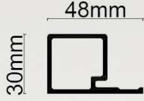
TRİO BAŞLANGIÇ PROFİLİ (PVC) TRİO START PROFILE (PVC)
