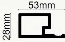
TERRA BAŞLANGIÇ PROFİLİ (WPC) TERRA START PROFILE (WPC)
